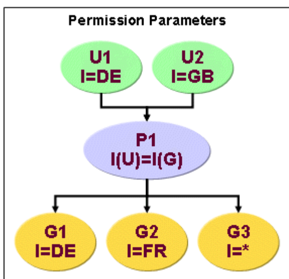
Figure 28. Example Permission Parameters
